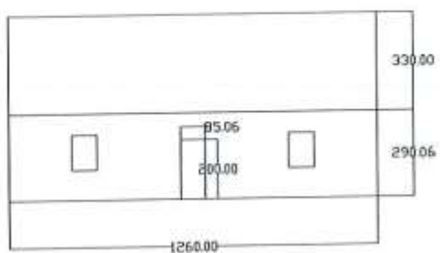
Elewacja wschodnia
