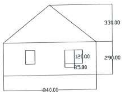
Elewacja północna
